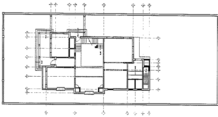
PLANTA BAJA - DEMONSTRACIONES Y MUROS NUEVOS DE 1/10
