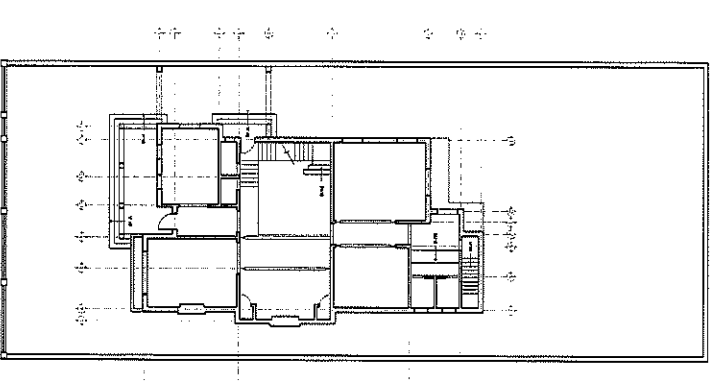
PLANTA BAJA - ESTADO ACTUAL DE 1/10
