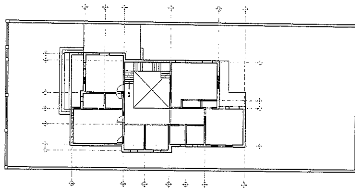
PLANTA ALTA - DEMONSTRACIONES Y MUROS NUEVOS DE 1/10
