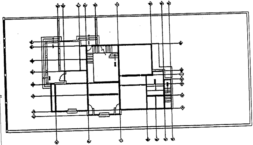
PLANTA BAJA
