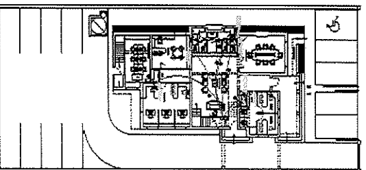
PLANTA BAJA
