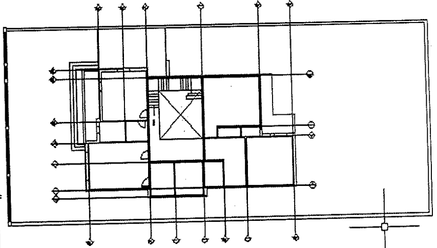
PLANTA ALTA
